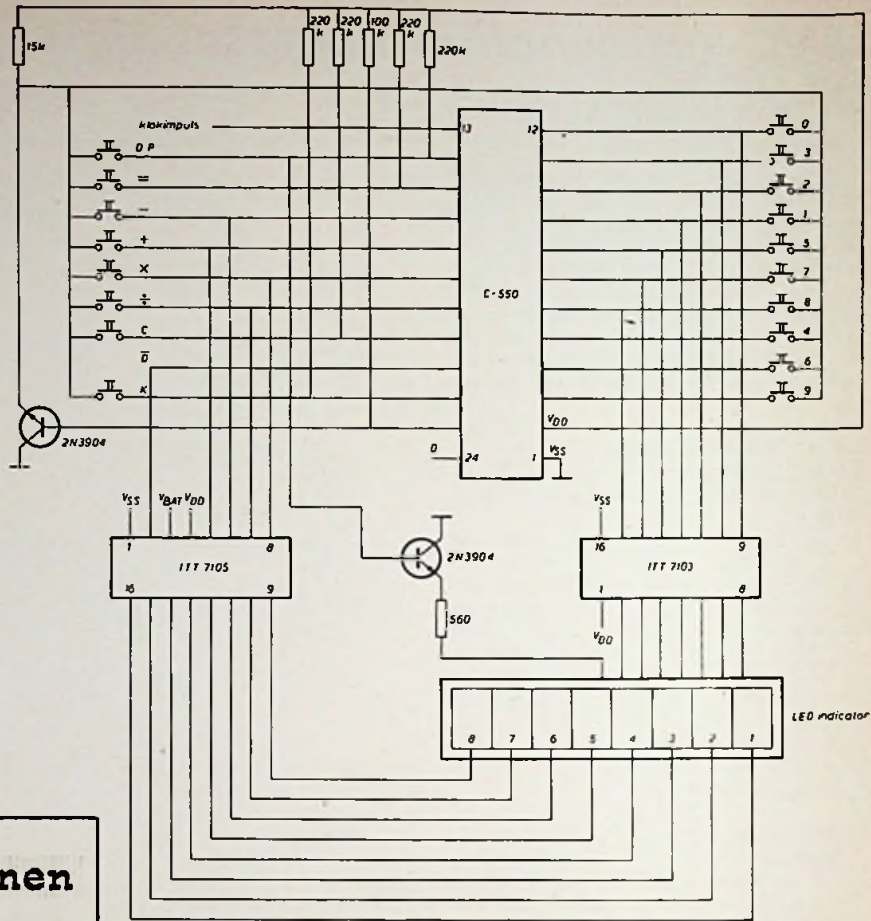
Fig. 1. De rekenchip C-550 met geïntegreerde stuurtrappen voor de LED-indicator.
